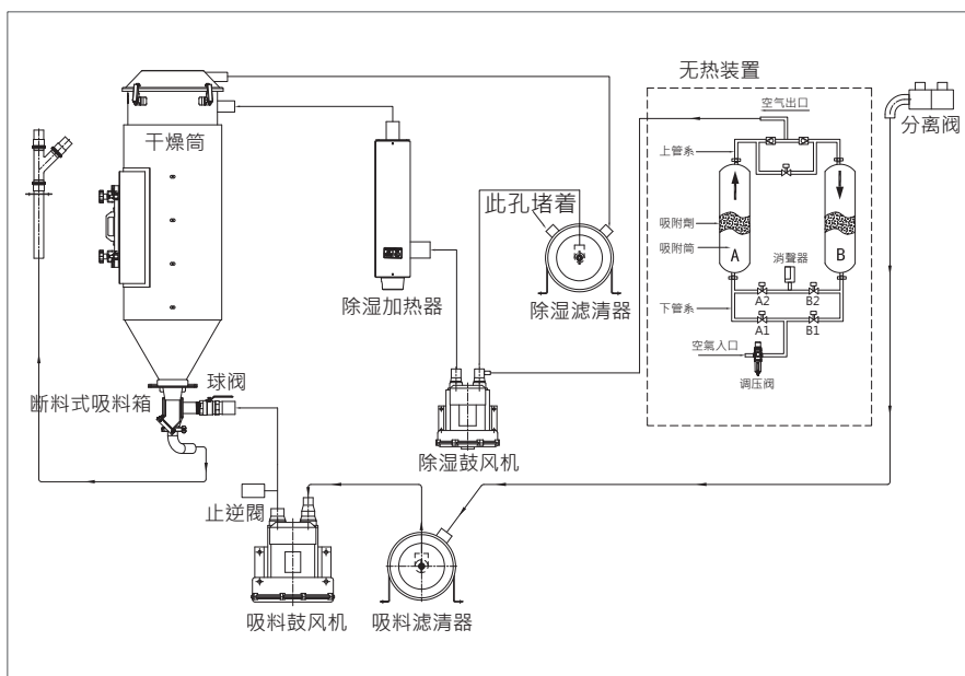
FCD-HL无热式工作原理图
