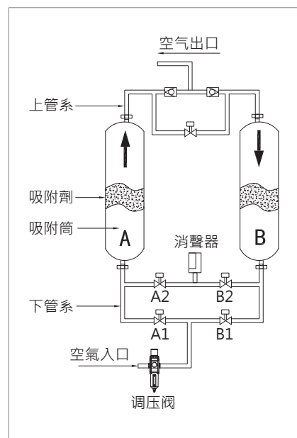
无热装置原理图
