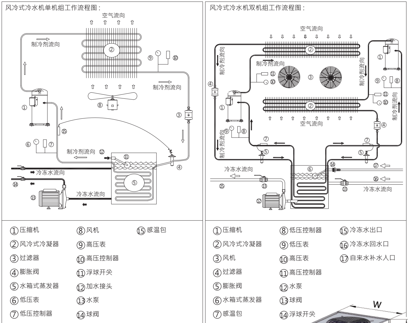
FAC风冷式冷水机
